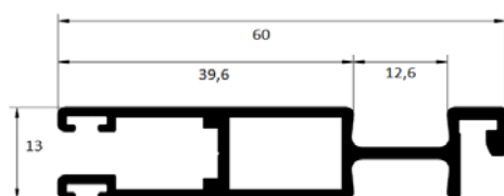
Wymiary: profil drzwi przesuwnych
