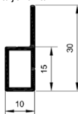
Wymiary: szyna jezdna "P"
