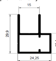
Wymiary: profil ramowy MPrz-2
